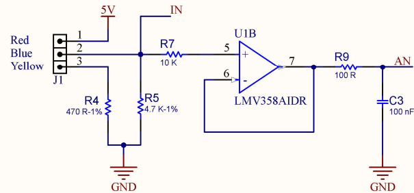
TSW-20M CIRCUIT
