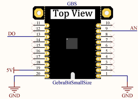
GEBRABIT PINOUT
